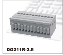
DG211R-2.5 160B/3A 0.2-0.5mm 2 150B/5A 28-20AWG Полосов 1P-XXP
