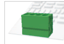
DG271V-7.5 1000B/41A 0.2-10.0mm 2 600B/40A 24-8AWG Полосов 1P-XXP
