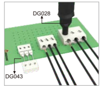
DG027 Переключатель DG028 Инструмент для демонтажа проводов
