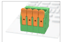
DG2204V-5.0 400B/32A 0.2-4.0mm 2 320B/20A 24-12AWG Полосов 1P-XXP
