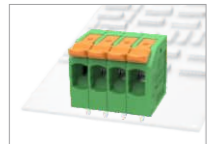
DG2204R-5.0 400B/32A 0.2-4.0mm 2 320B/20A 24-12AWG Полосов 1P-XXP
